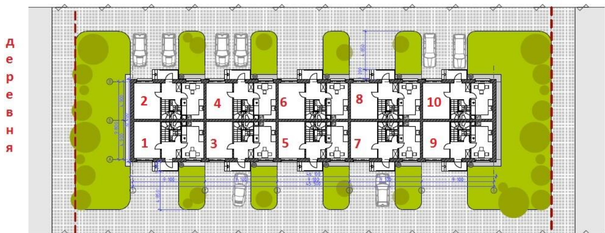
План 1-го этажа здания, генплан придомовой территории.
